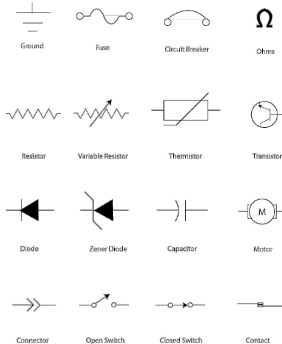
Elektrische Symbolen
